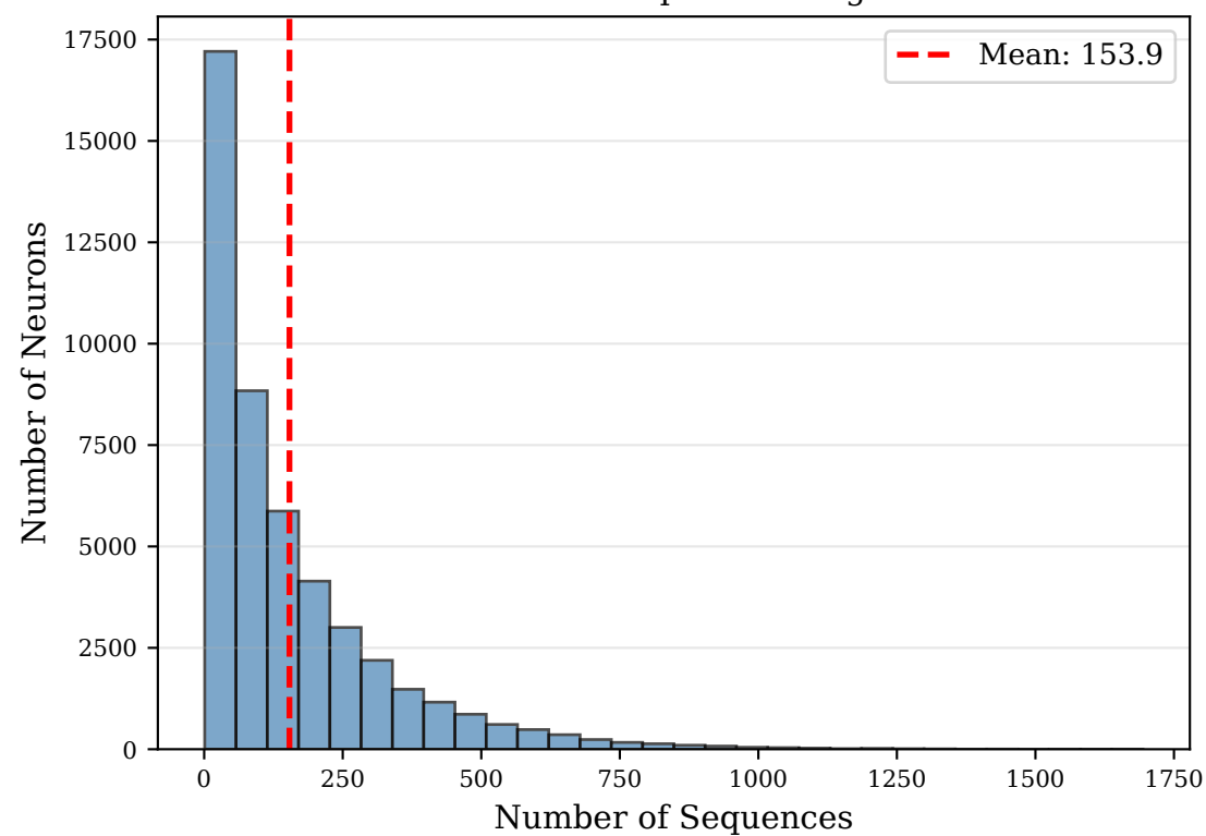
Neuron Participation - Original
